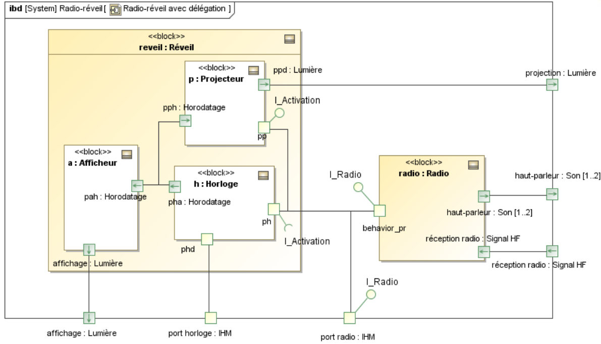
Le diagramme de bloc interne « ibd »
