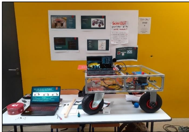
Lycée Couffignal: Terminale STI2D Chariot mobile suiveur
