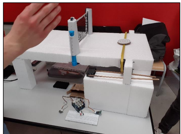
Lycée Don Bosco: Première SI Table de tennis connectée
